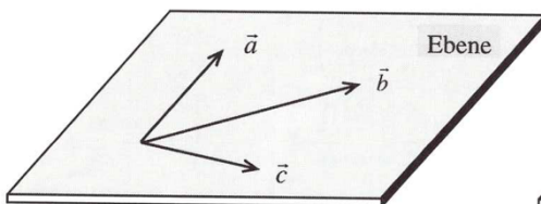
komplanare Vektoren
